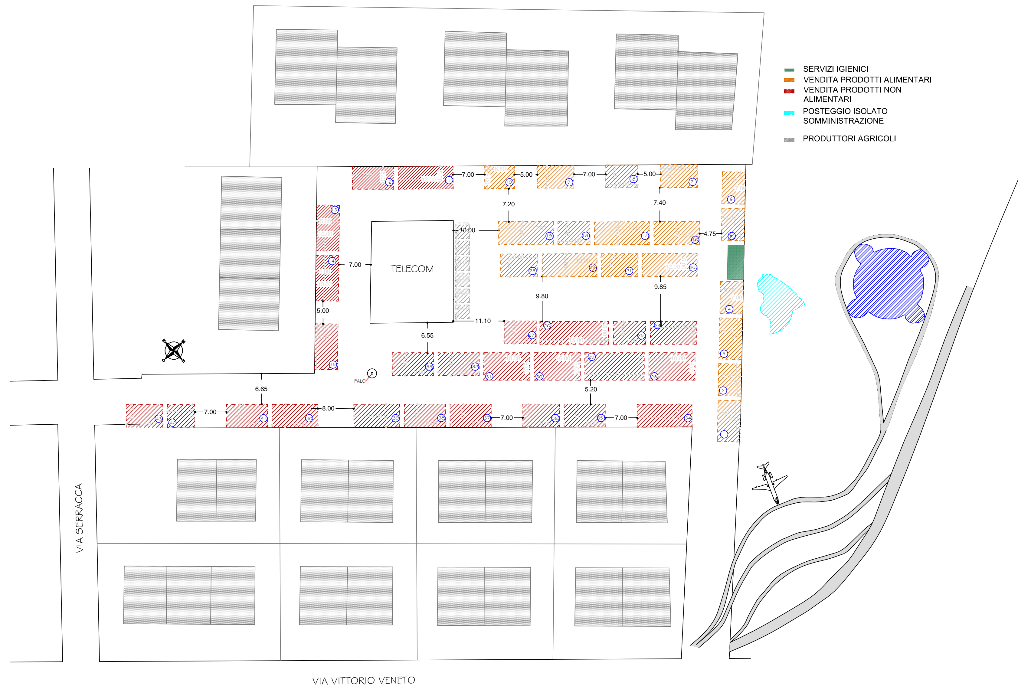
PLANIMETRIA — scala 1:500 —
